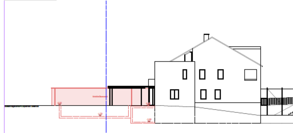
Ansicht Südost
