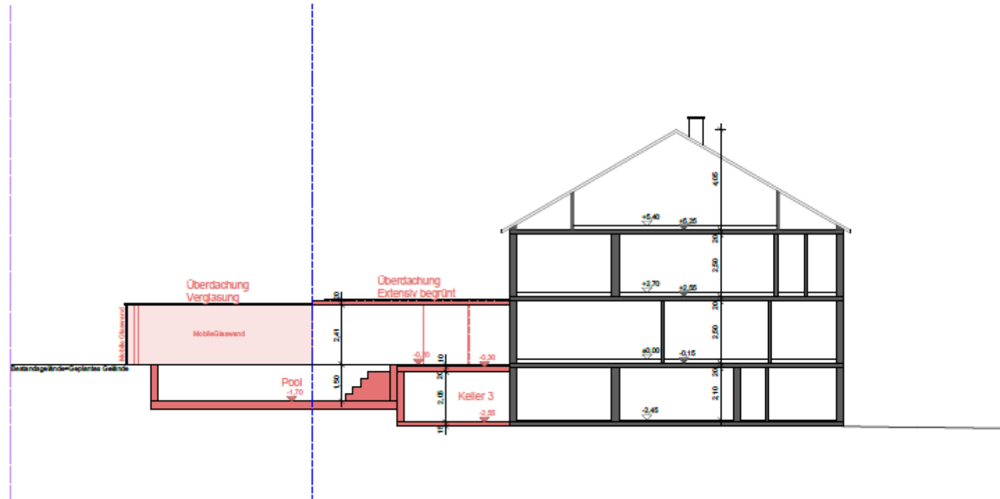
Schnitt A-A
